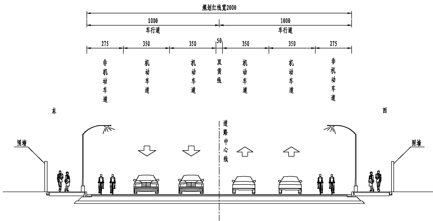
道路标准横断面图
