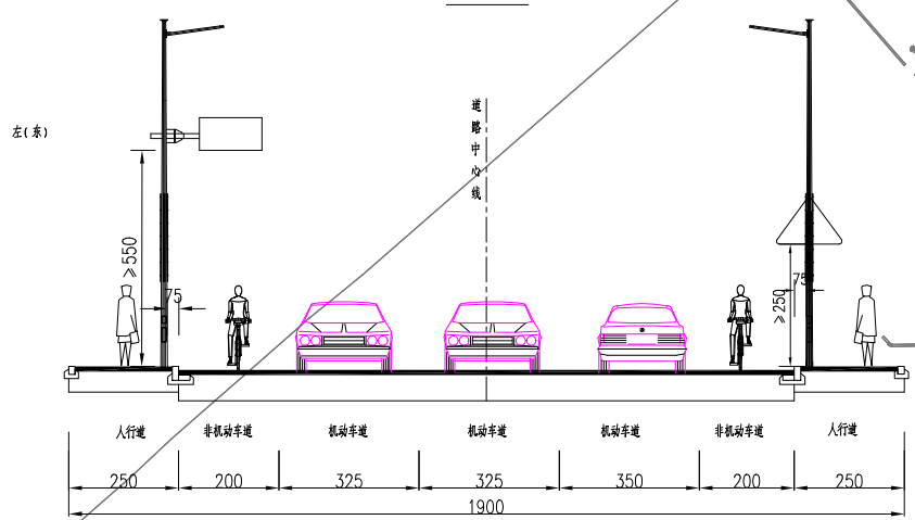
道路标准横断面
