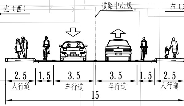
堰桥路标准横断面图
