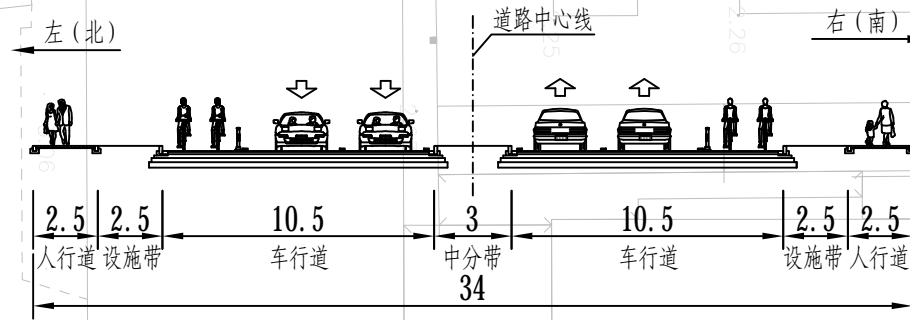
堰新路标准横断面图
