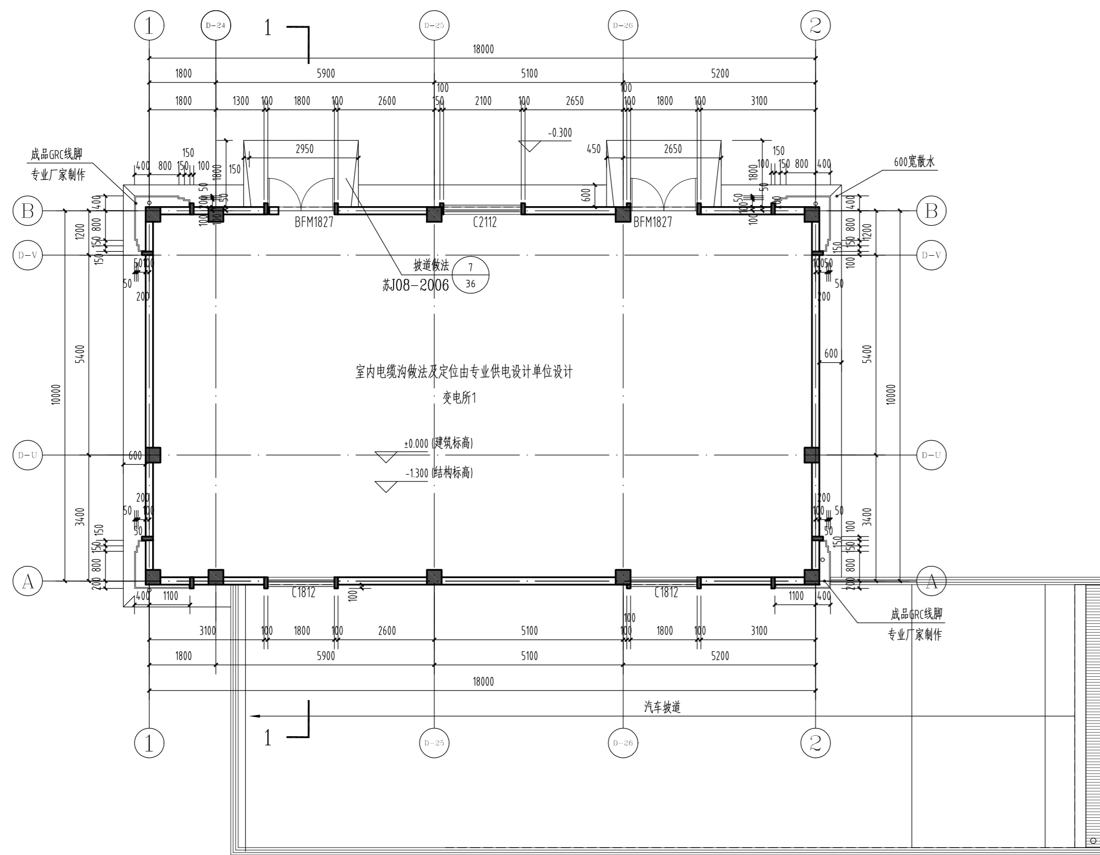
一层平面图 1:100
