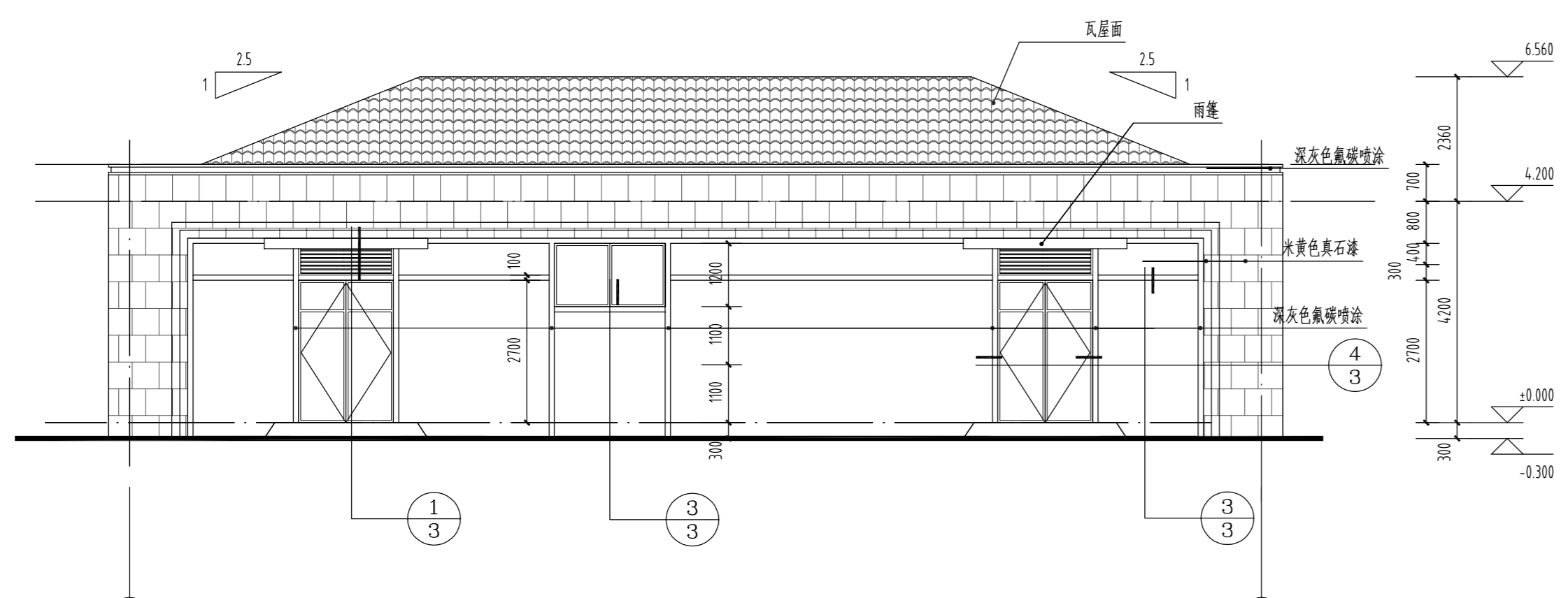
变电所1②~①立面图 1:100
