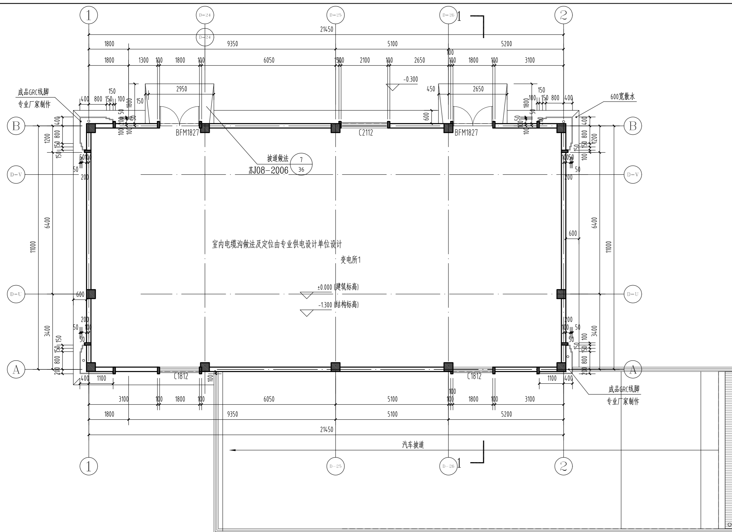
一层平面图 1:100
