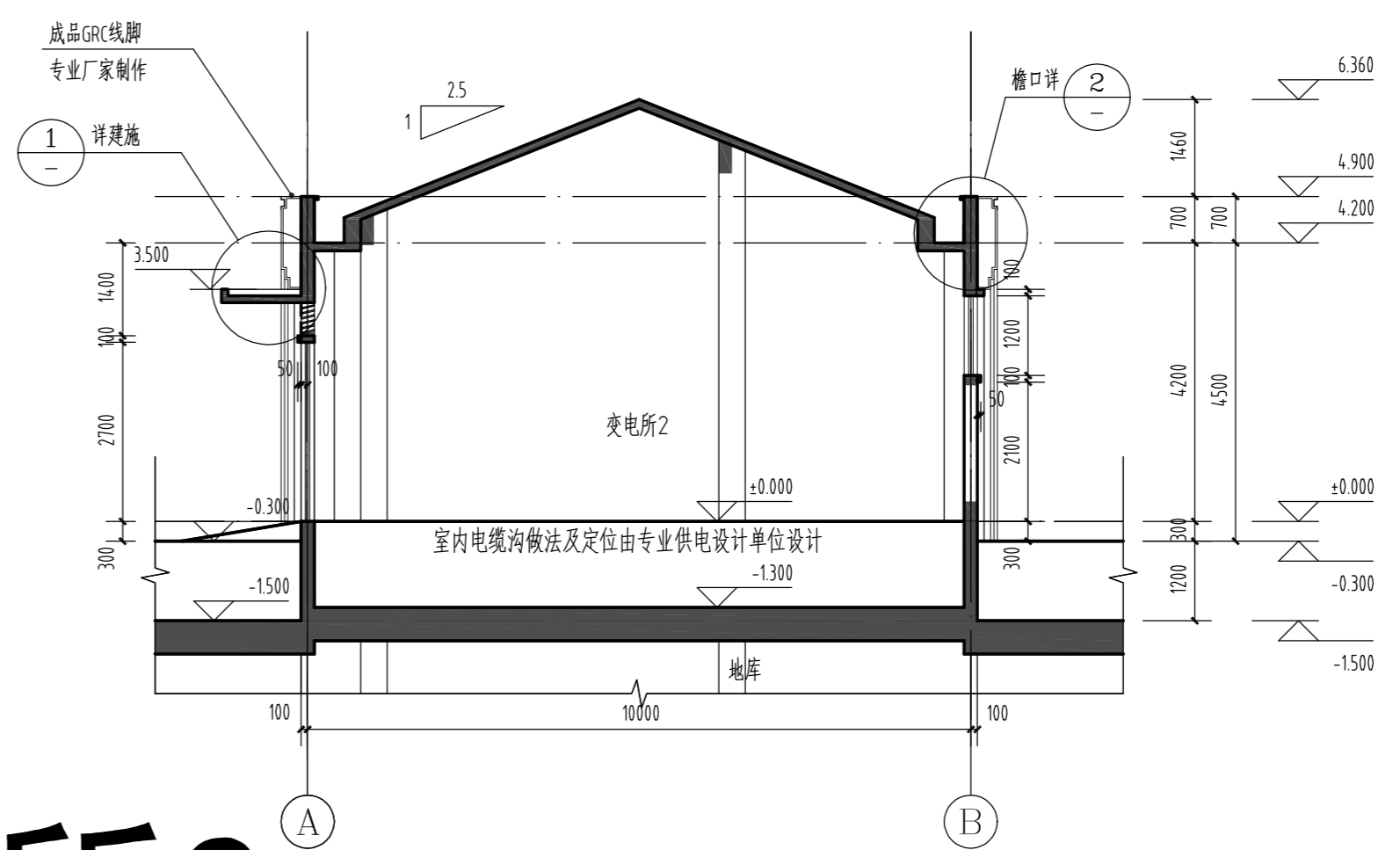
变电所2 2-2剖面图 1:100
