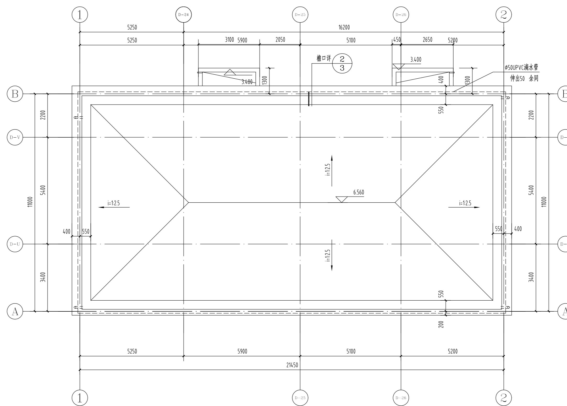
屋顶平面图 1:100
