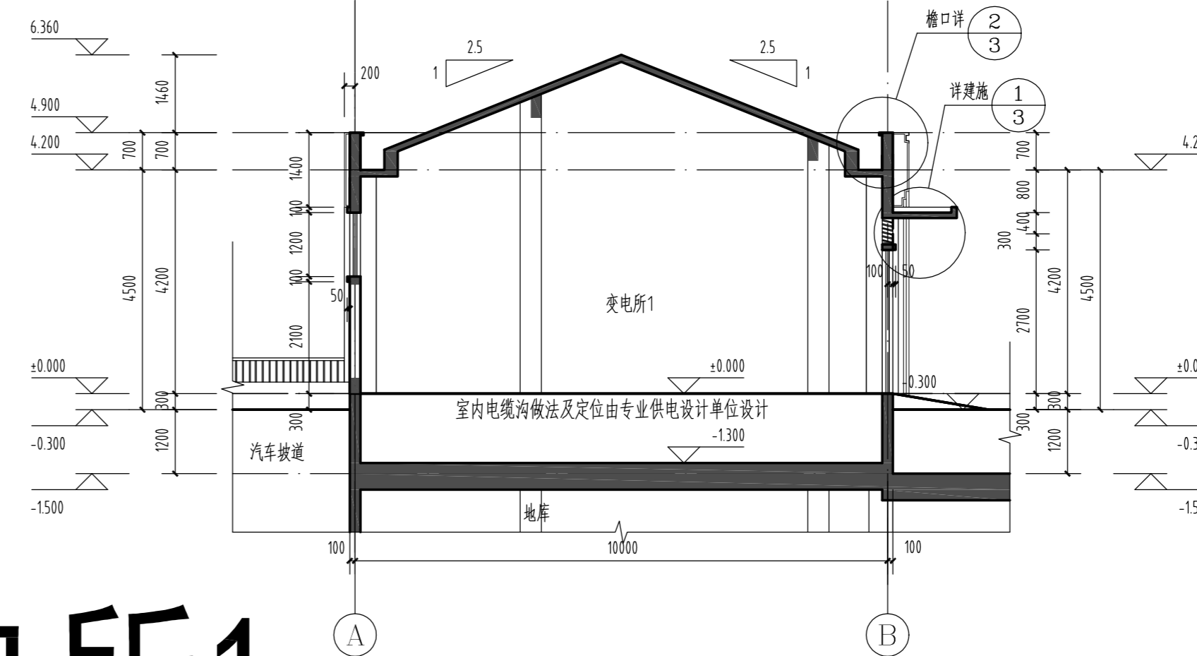
变电所1 1-1剖面图 1:100
