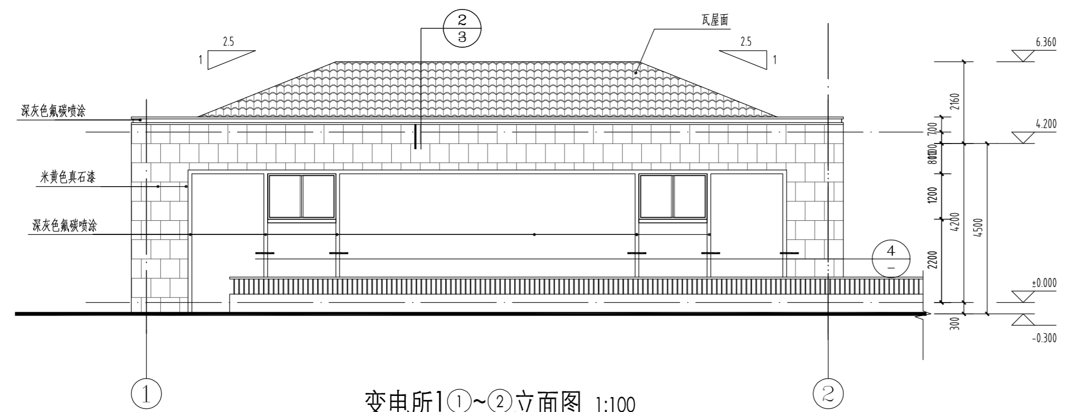
变电所1①~②立面图 1:100
