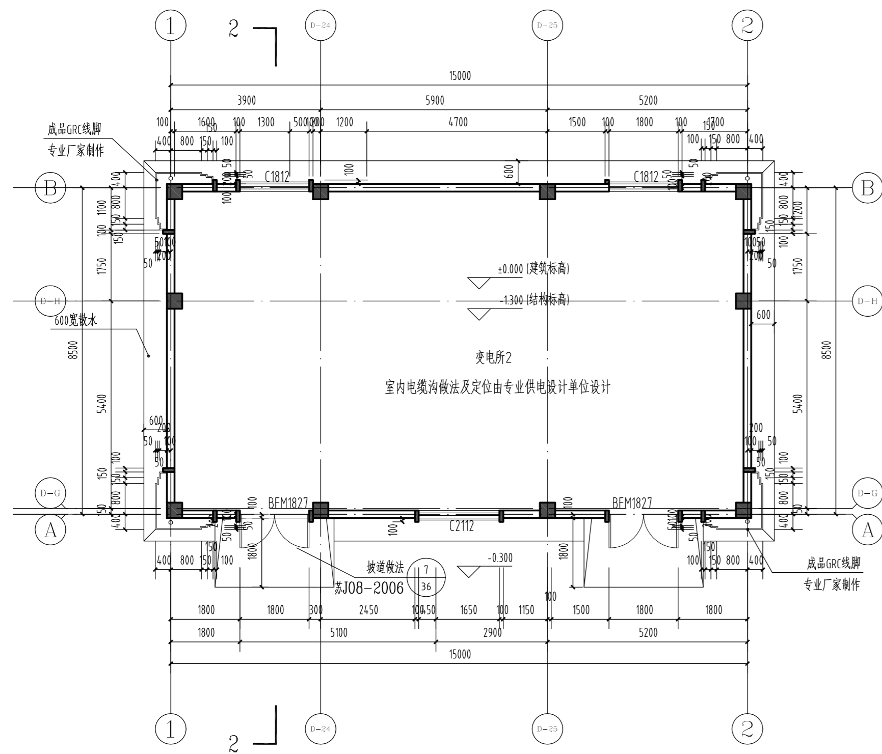
一层平面图 1:100
